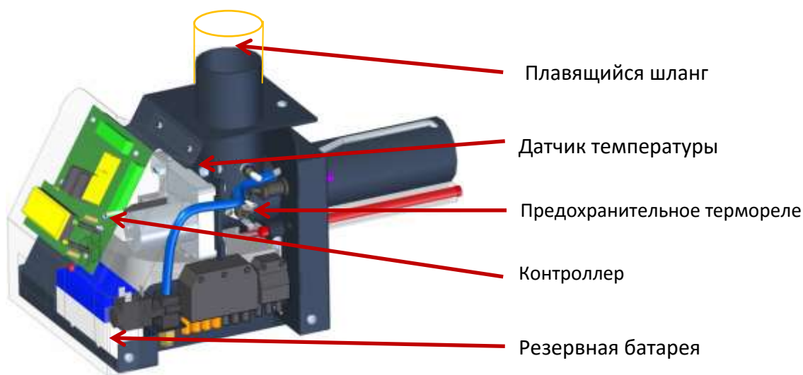
Рисунок 2 Устройства безопасности
