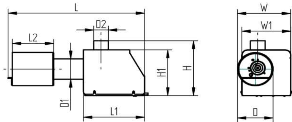
Рисунок 3 Основные размеры
