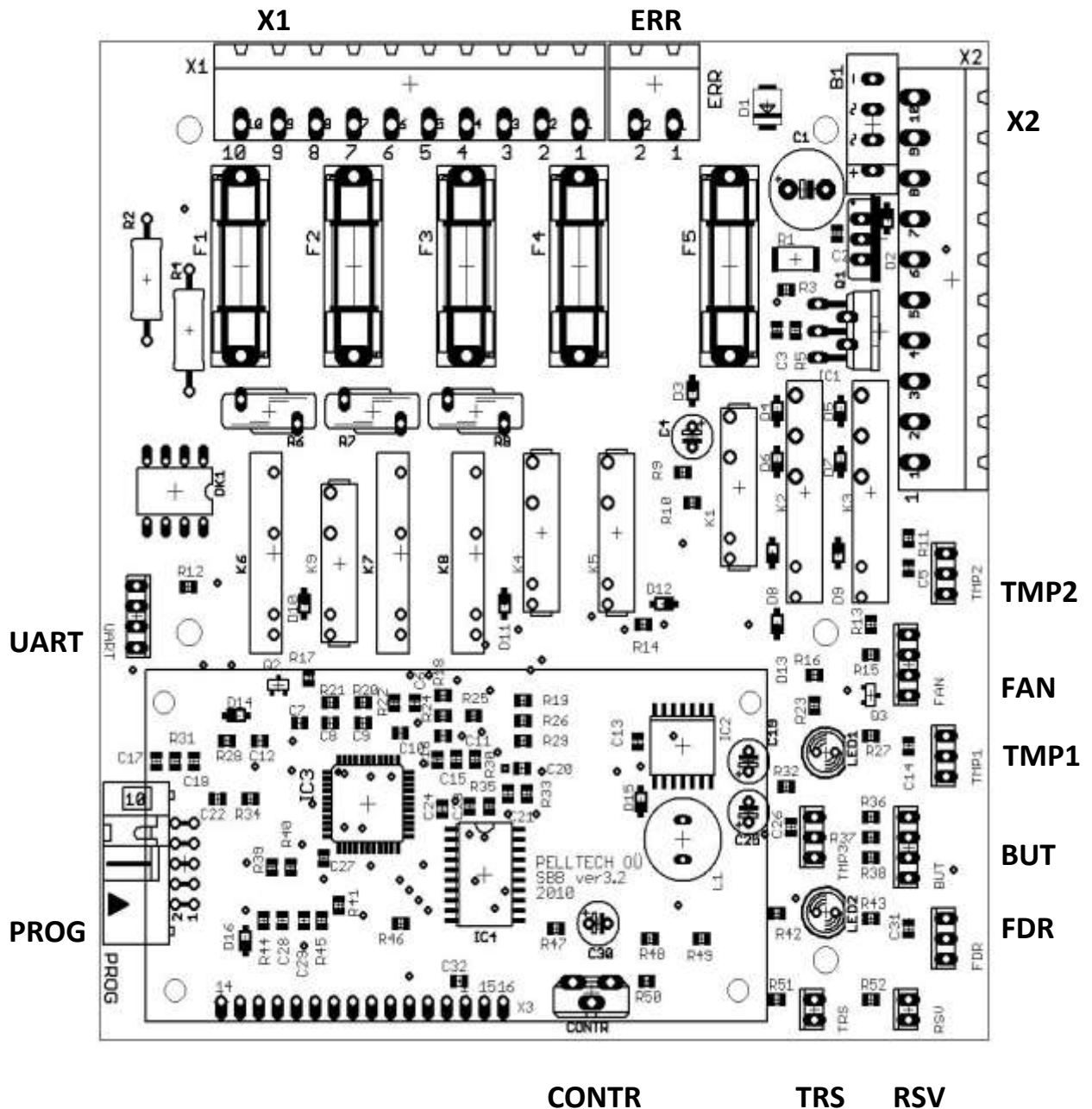
Рисунок 23 Контроллер SBB 3.2
