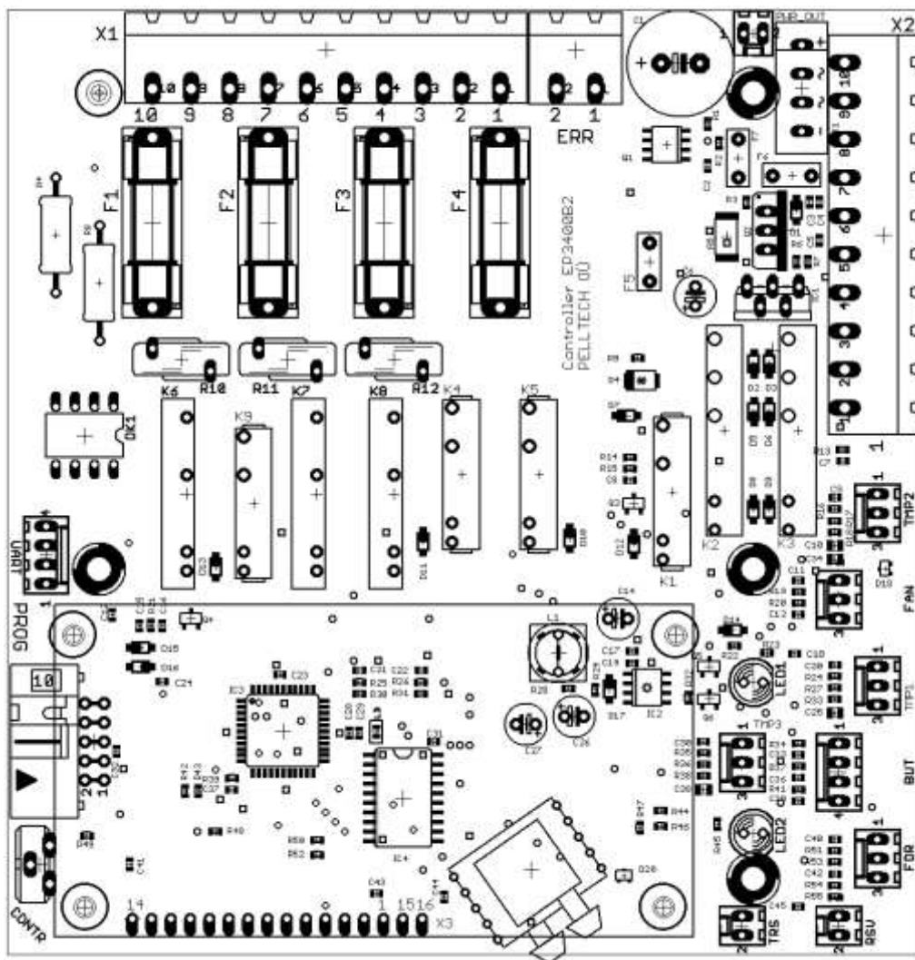
Рисунок 24 Контроллер EP3200A1
